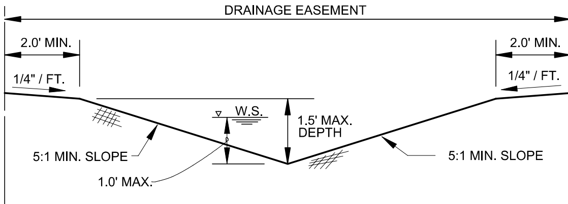
"V" - SHAPED CHANNEL N.T.S.
